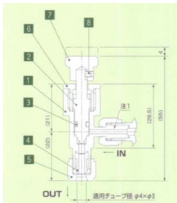
剖面尺寸圖
